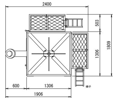
サイロ姿図
